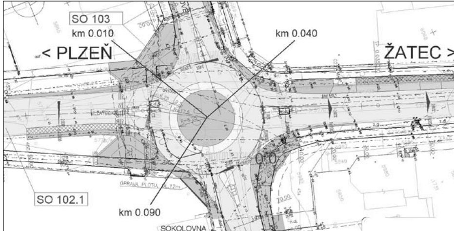
Projekt kruhového objezdu na silnici č. 27 u sokolovny
